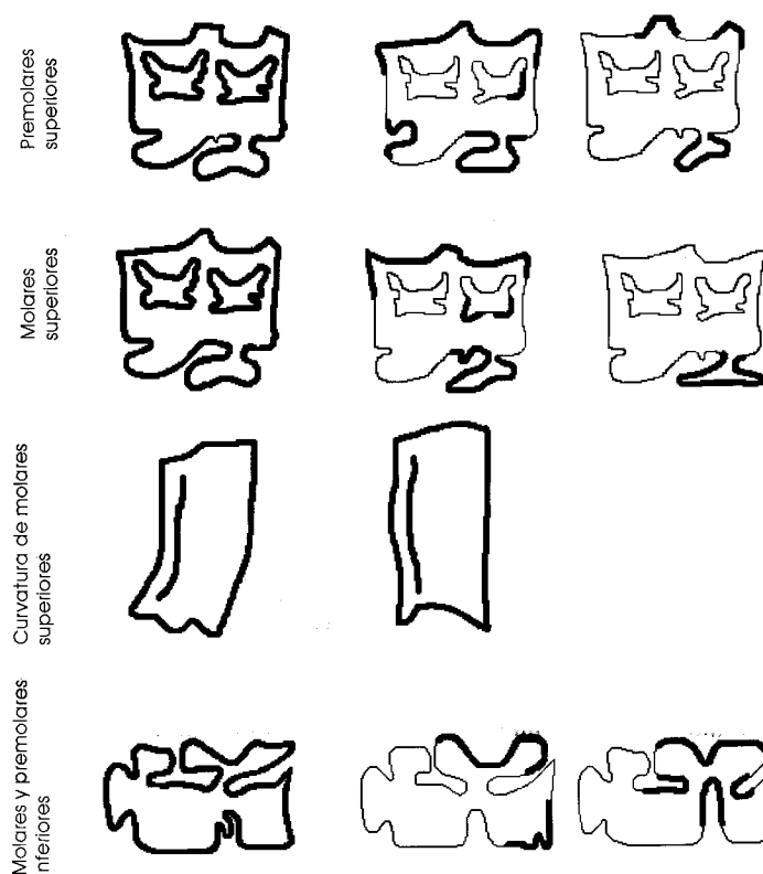
Figura 13.- Forma en los patrones dentales comunes y poco frecuentes en molares y premolares (a) superiores y (b) inferiores.
