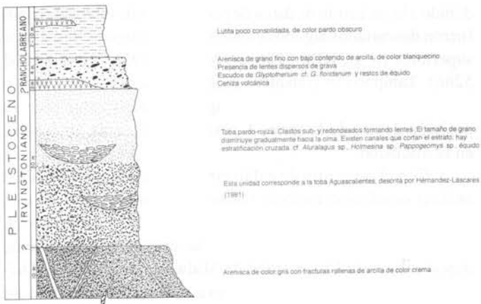
Figura 3.- Columna estratigráfica del área de estudio.
